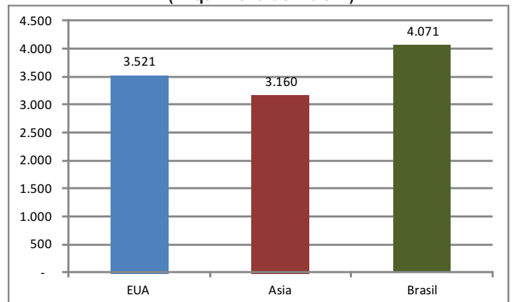
Comparativo do preço do PEBDL nacional e preços Spot de mercados de referência internados* (2ª quinzena de mar/12)
