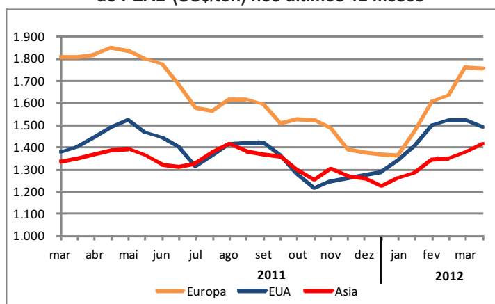
Comportamento dos preços SPOT nos mercados referência do PEAD (US$/ton) nos últimos 12 meses
