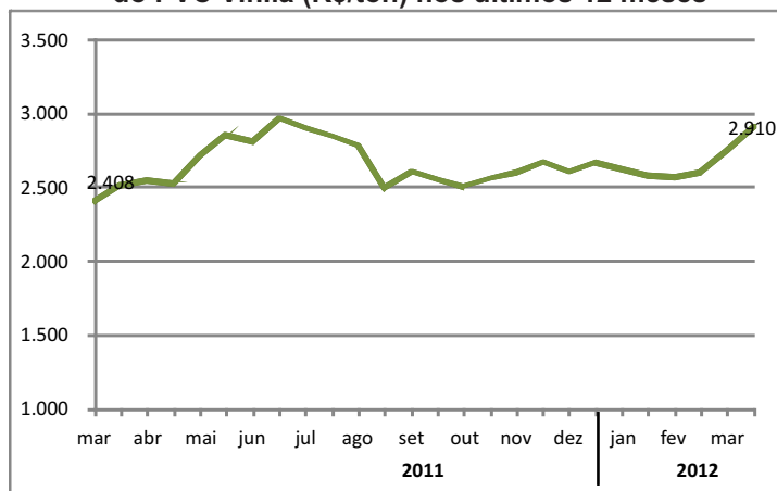
Comportamento dos preços domésticos brasileiros do PVC Vinila (R$/ton) nos últimos 12 meses
